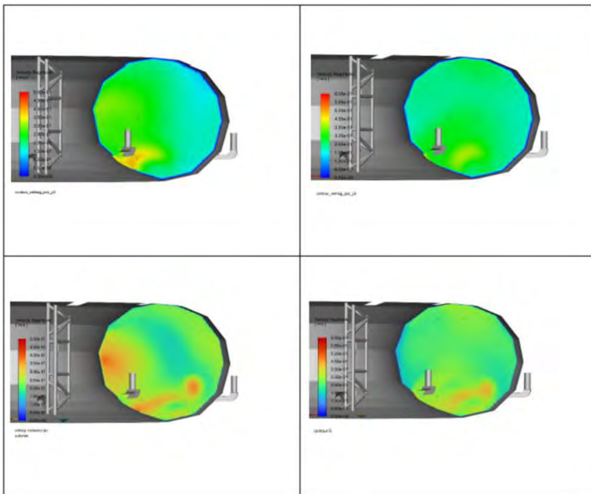
Figur 12 Hastigheter i måleplanet ved luke 6 (mellom strømsettere). Øvre, venstre: Original plassering av mikserne, 60% modus. Øvre, høyre: Original plassering, 100% modus. Nedre venstre: Senket posisjon, 60% modus. Nedre, høyre: Senket posisjon, 100% modus.
